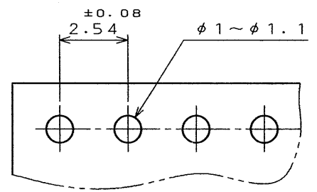
基板取付寸法 (尺度5:1)
