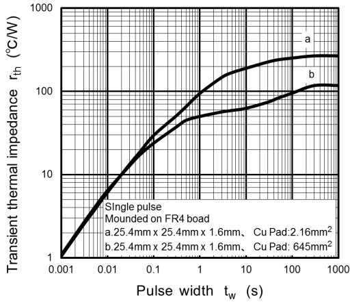
Fig. 7.13 r_{th} - t_w
