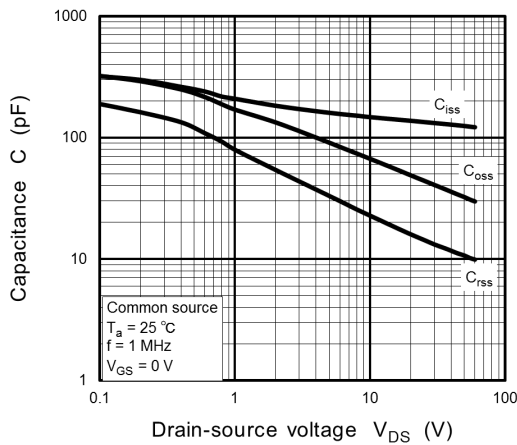
Fig. 7.11 C - V_{DS}
