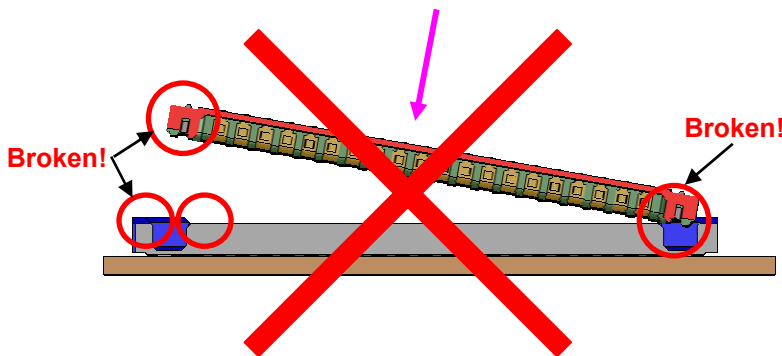
コネクタ斜め嵌合 Mating with angle (Wrong Handling)
