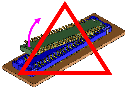
長手方向の斜め抜去
