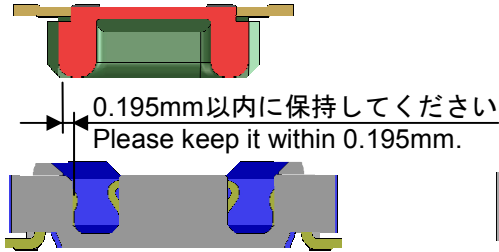
短手方向 "b" Direction
