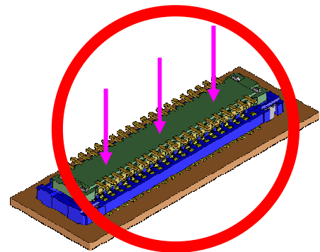
コネクタ全体 平行押し込み Pushing Whole Paralleled (Correct Handling)
