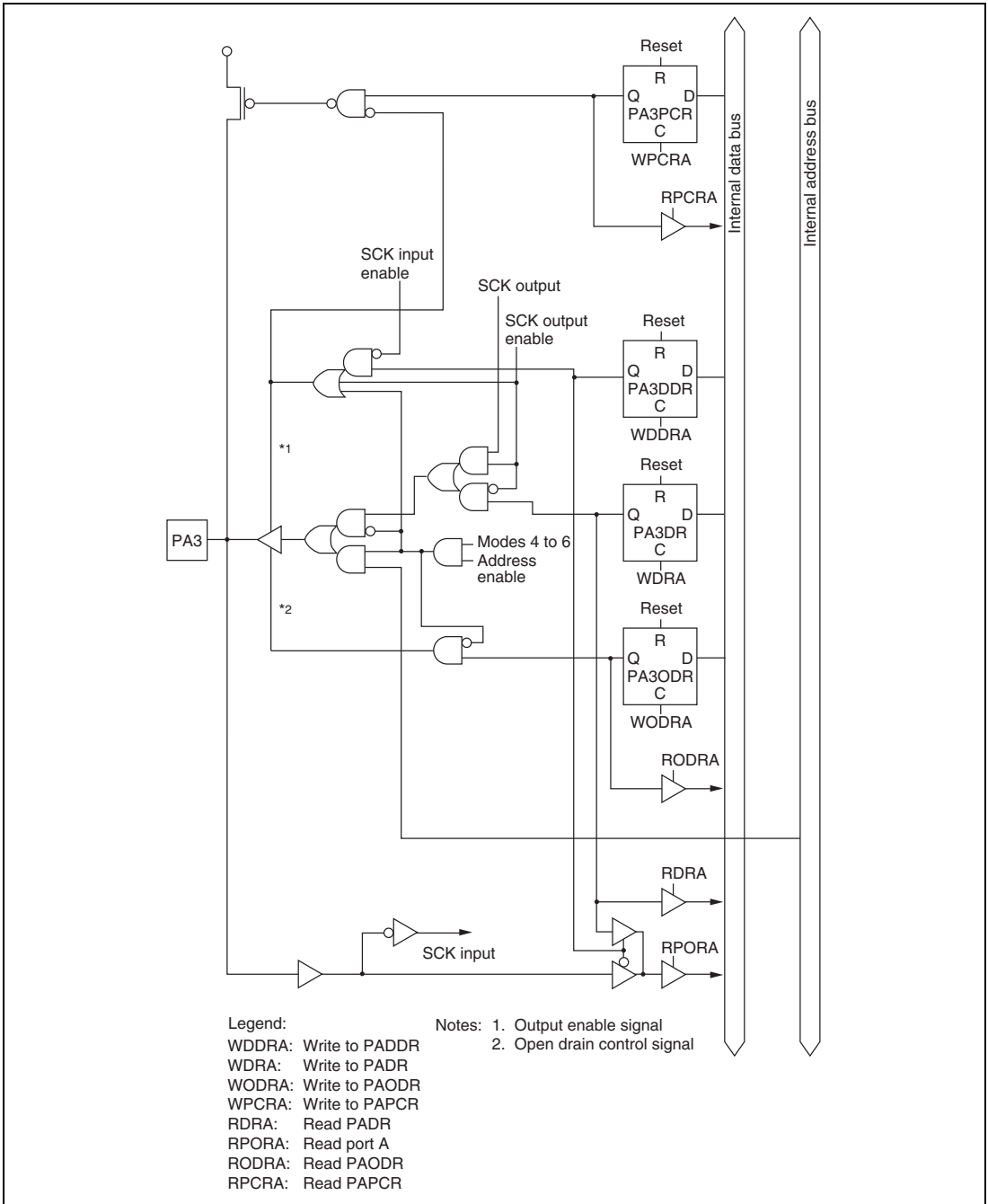
Figure C.6 (d) Port A Block Diagram (Pin PA3)
